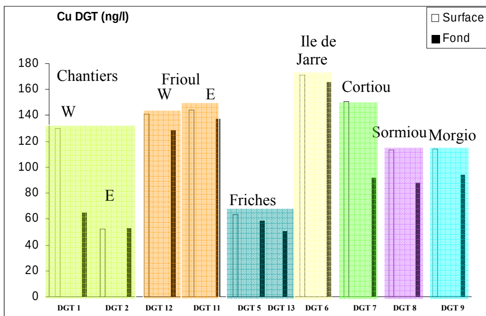
Figure 21 : Profil des concentrations en cuivre mesurées par les DGT
