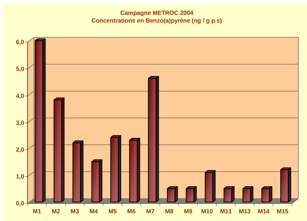
Figure 31: Profil des concentrations en benzo(a)pyrène mesurées dans les moules
