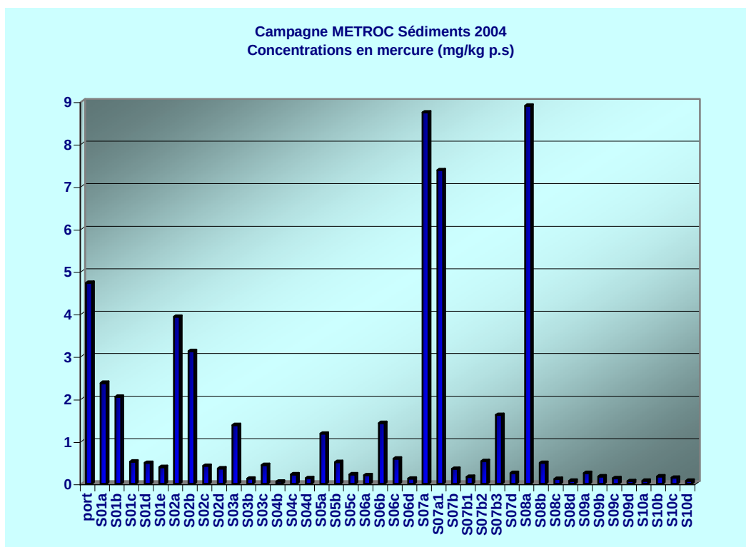
Figure 13 : Profil des concentrations en mercure mesurées dans les sédiments
