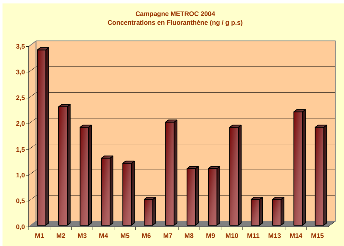
Figure 23 : Profil des concentrations en Fluoranthène mesurées dans les moules.
