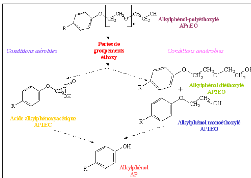
Figure 50 : Schéma de principe du phénomène de biodégradation des APnEO
