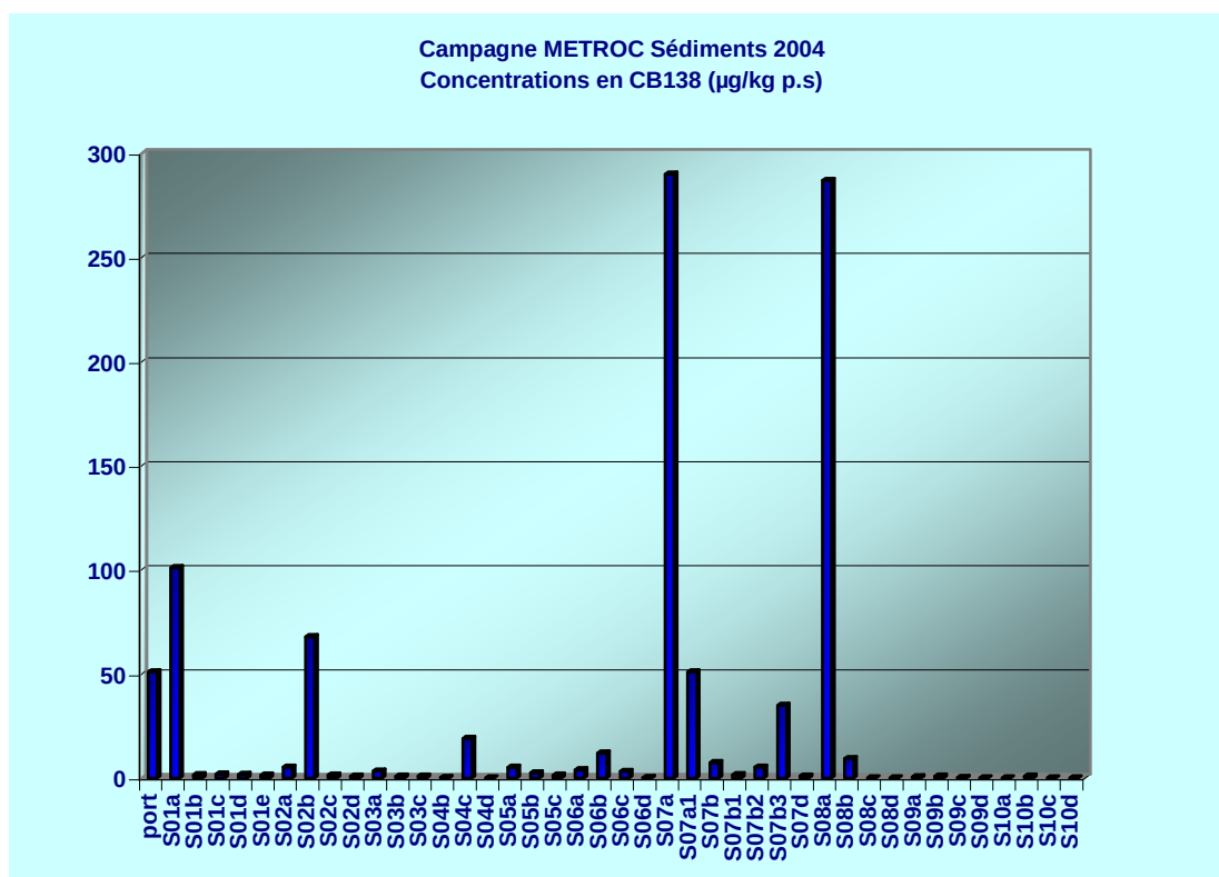
Figure 42 : Profil des concentrations en CB138 mesurées dans les sédiments
