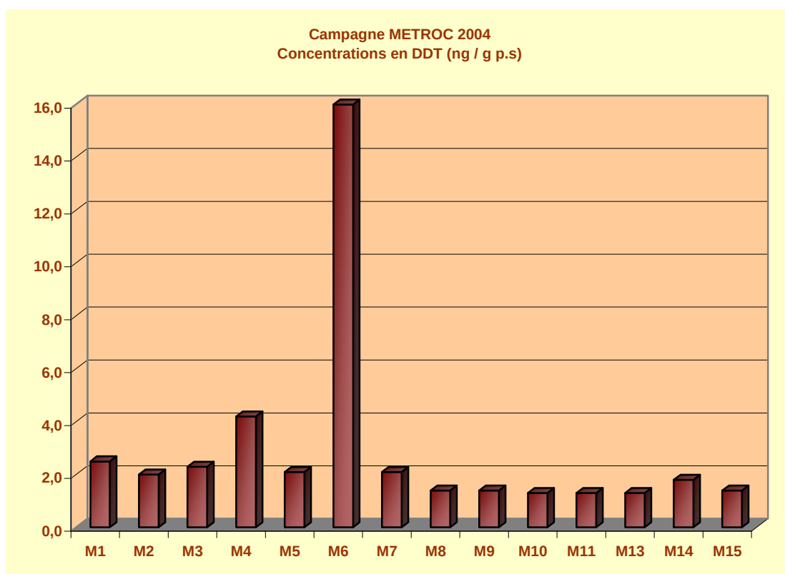
Figure 37 : Profil des concentrations en DDT mesurées dans le biote
