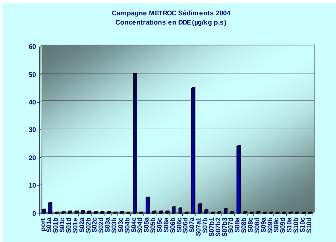
Figure 38 : Profil des concentrations en DDE mesurées dans les sédiments
