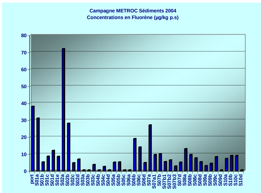
Figure 26 : Profil des concentrations en Fluorène mesurées dans les sédiments
