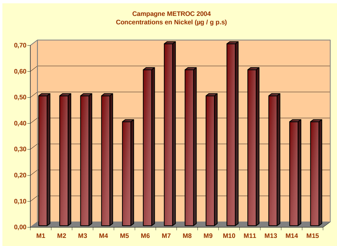
Figure 16 : Profil des concentrations en nickel mesurées dans le biote (cf carte 6 vol 2)
