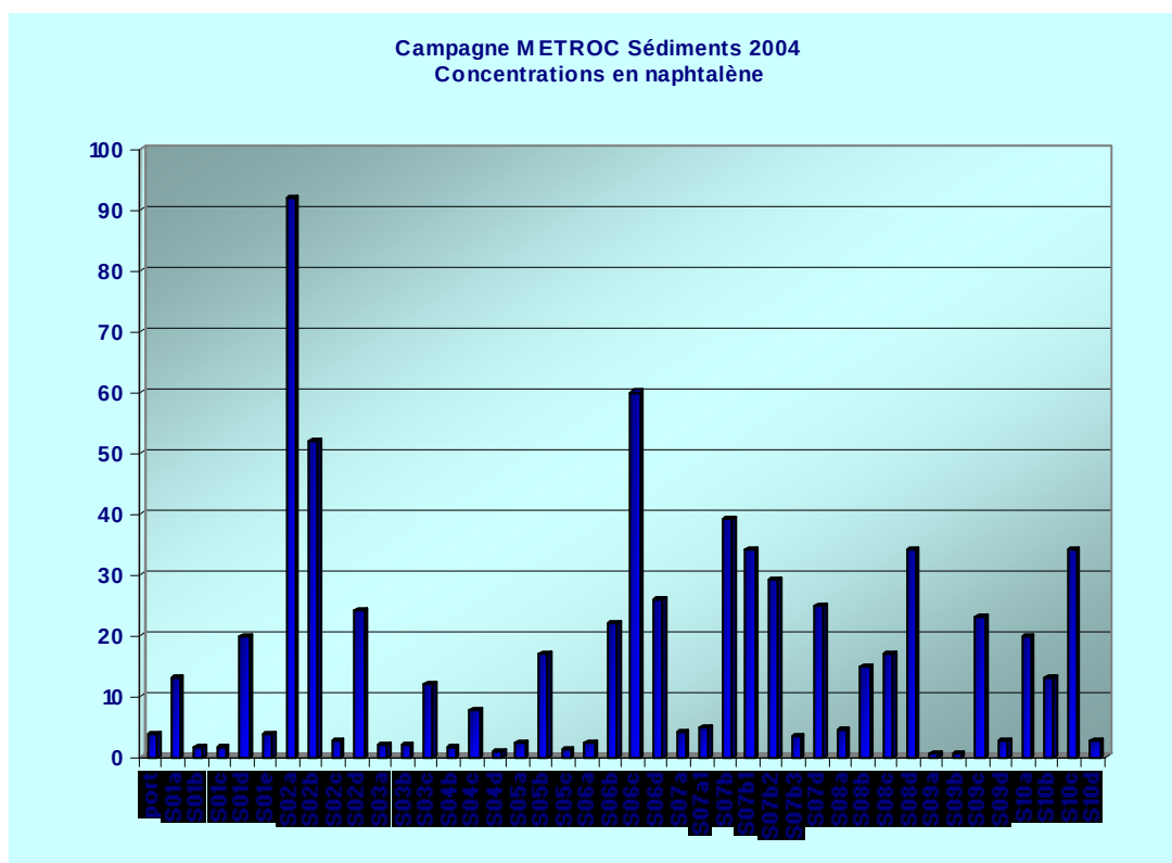
Figure 24 : Profil des concentrations en naphtalène mesurées dans les sédiments
