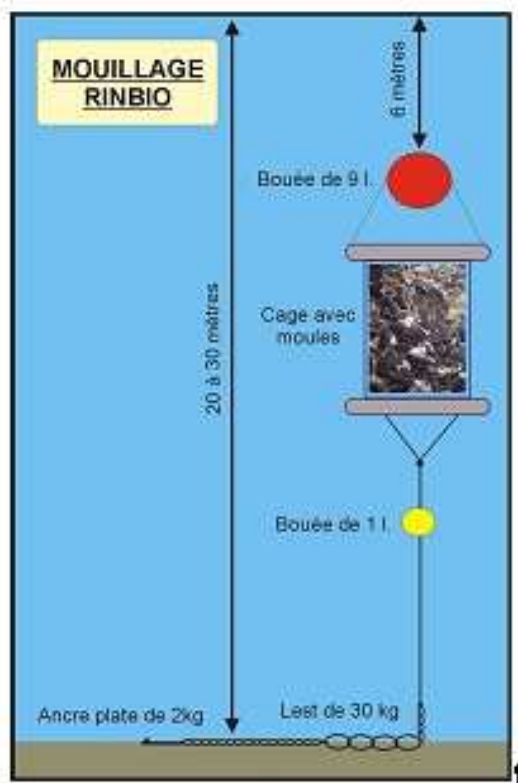
Figure 5 : Schéma de mouillage RINBIO
