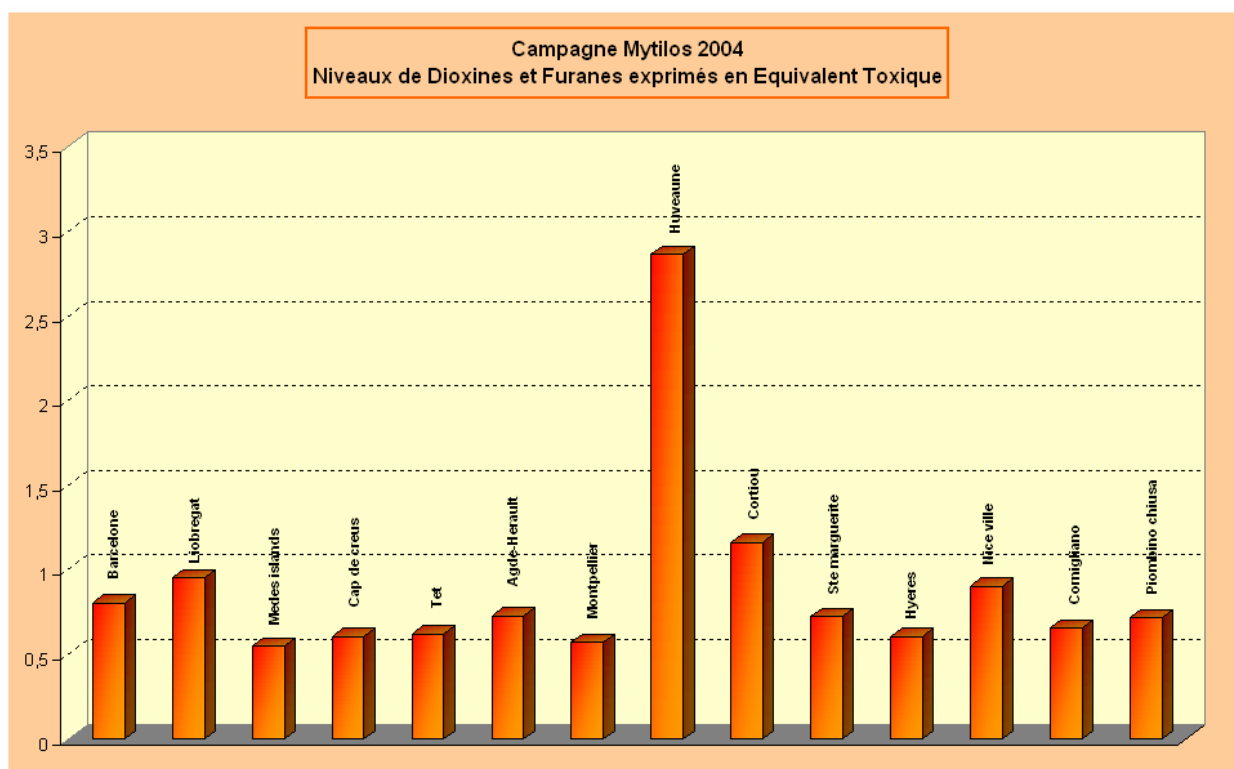
Figure 48 : Campagne MYTILOS 2004, contamination par les dioxines et furanes (en pg/g p. s.)
