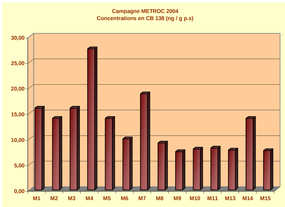
Figure 43 : Profil des concentrations en CB138 mesurées dans le biote
