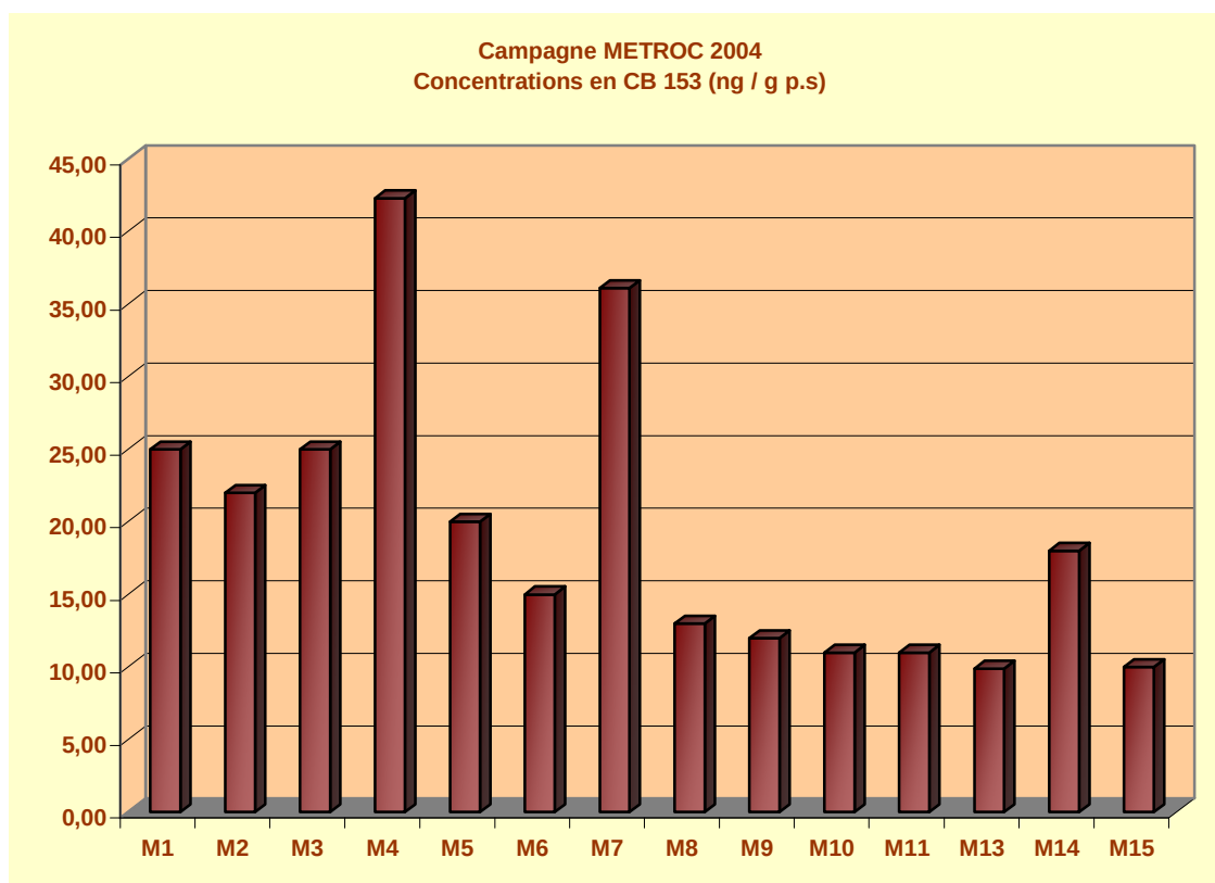
Figure 45 : Profil des concentrations en CB153 mesurées dans le biote
