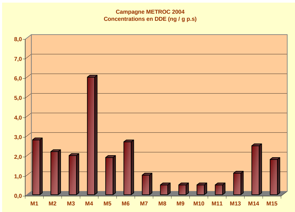
Figure 39 : Profil des concentrations en DDE mesurées dans le biote
