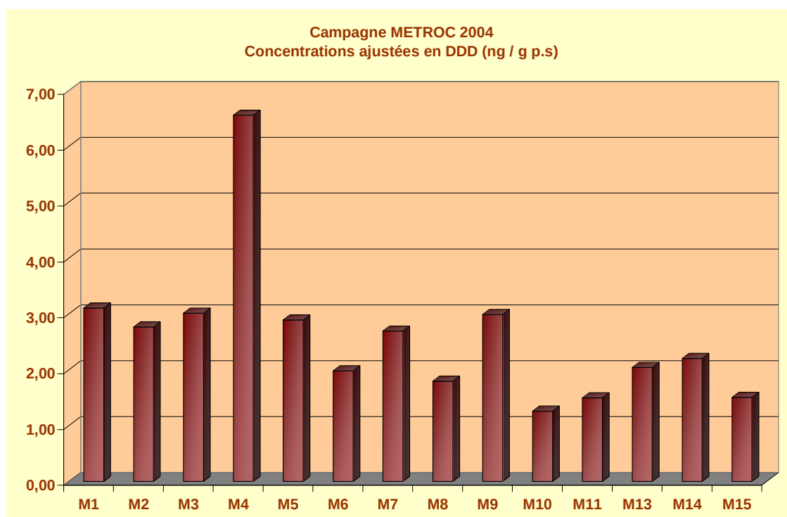
Figure 41 : Profil des concentrations en DDD mesurées dans le biote
