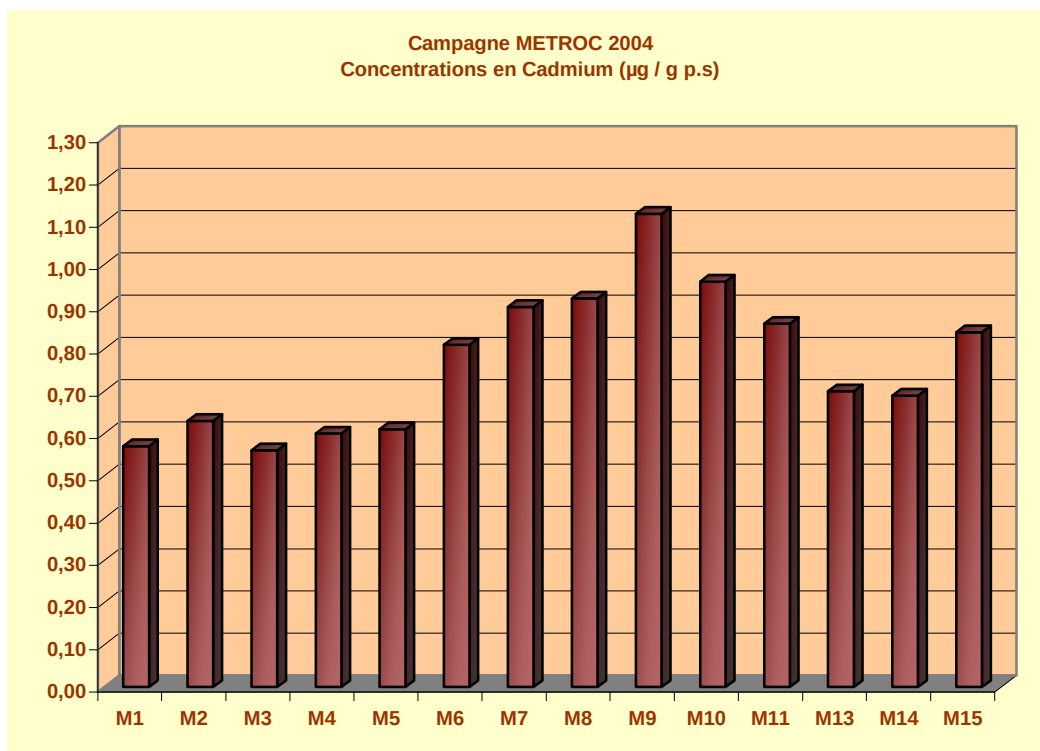
Figure 11 : Profil des concentrations en cadmium mesurées dans le biote.
