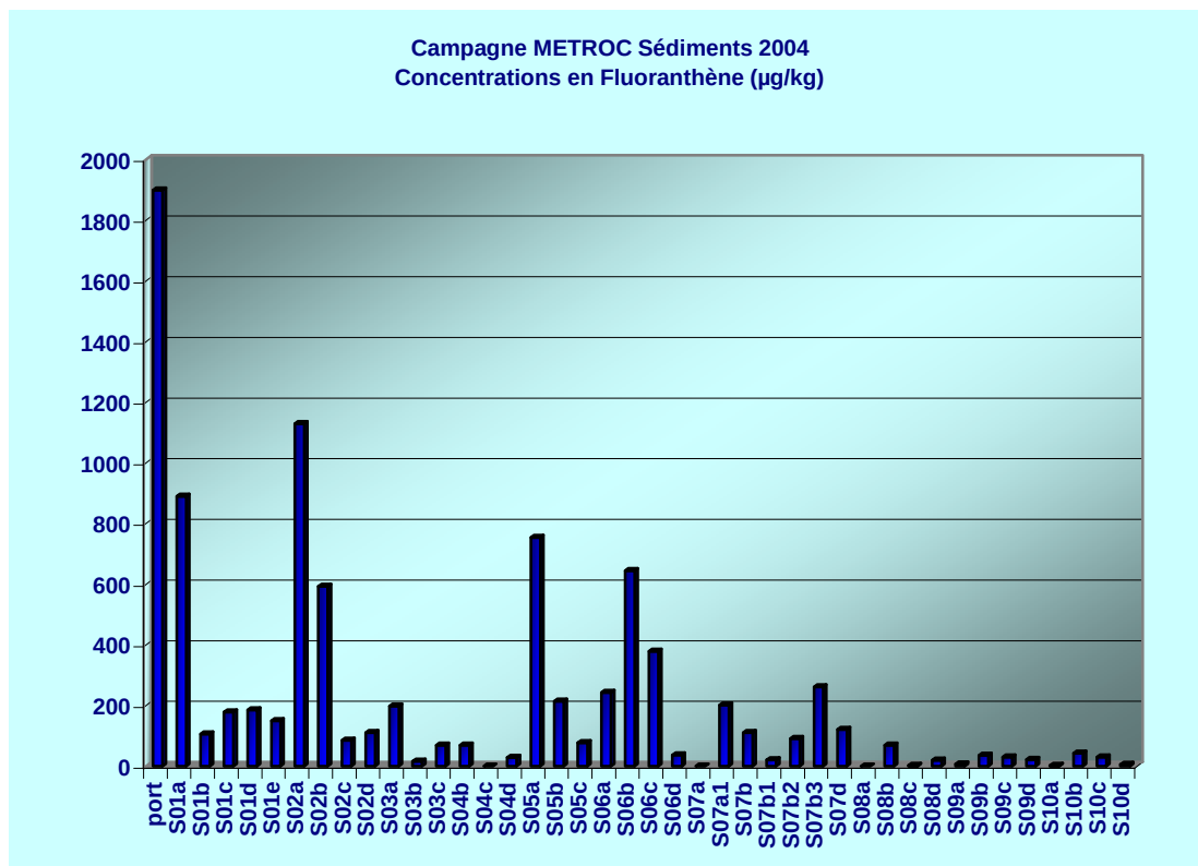
Figure 22 : Profil des concentrations en Fluoranthène mesurées dans les sédiments
