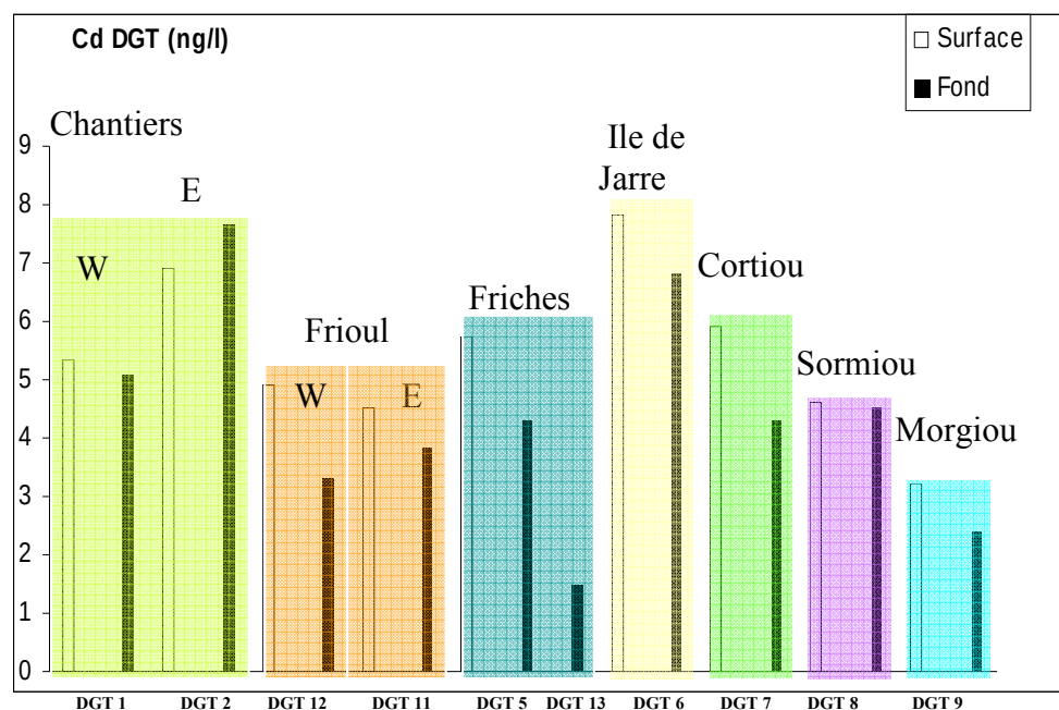
Figure 12 : Profil des concentrations en cadmium mesurées par les DGT
