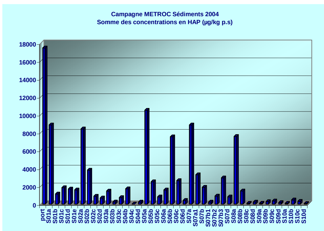
Figure 34 : Profil des concentrations de la somme des HAP mesurées dans les sédiments
