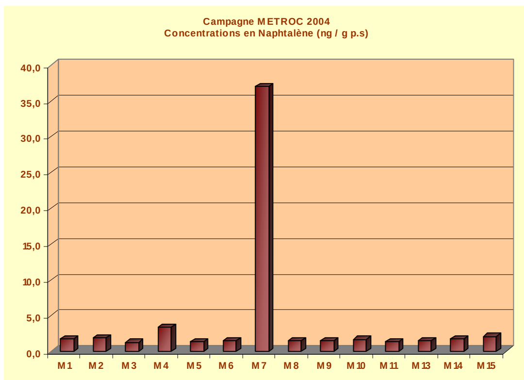
Figure 25 : Profil des concentrations en naphtalène mesurées dans le biote
