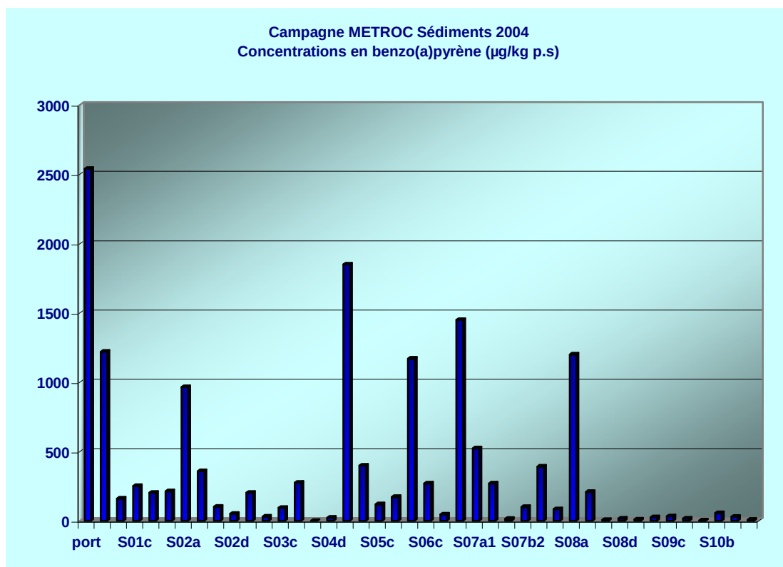
Figure 30 : Profil des concentrations en benzo(a)pyrène mesurées dans les sédiments
