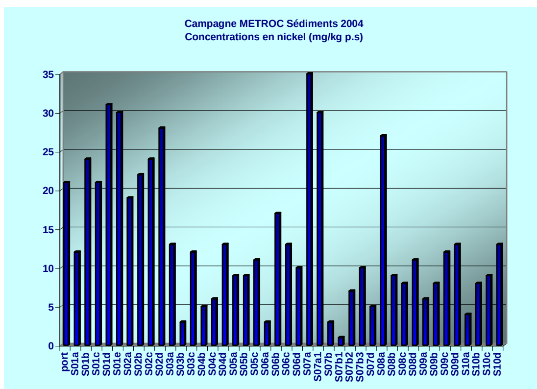
Figure 15 : Profil des concentrations en nickel mesurées dans les sédiments
