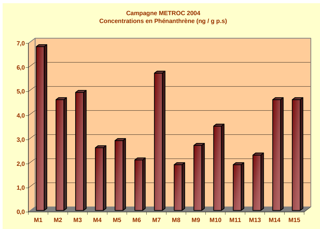
Figure 29 : Profil des concentrations en Phénanthrène mesurées dans le biote
