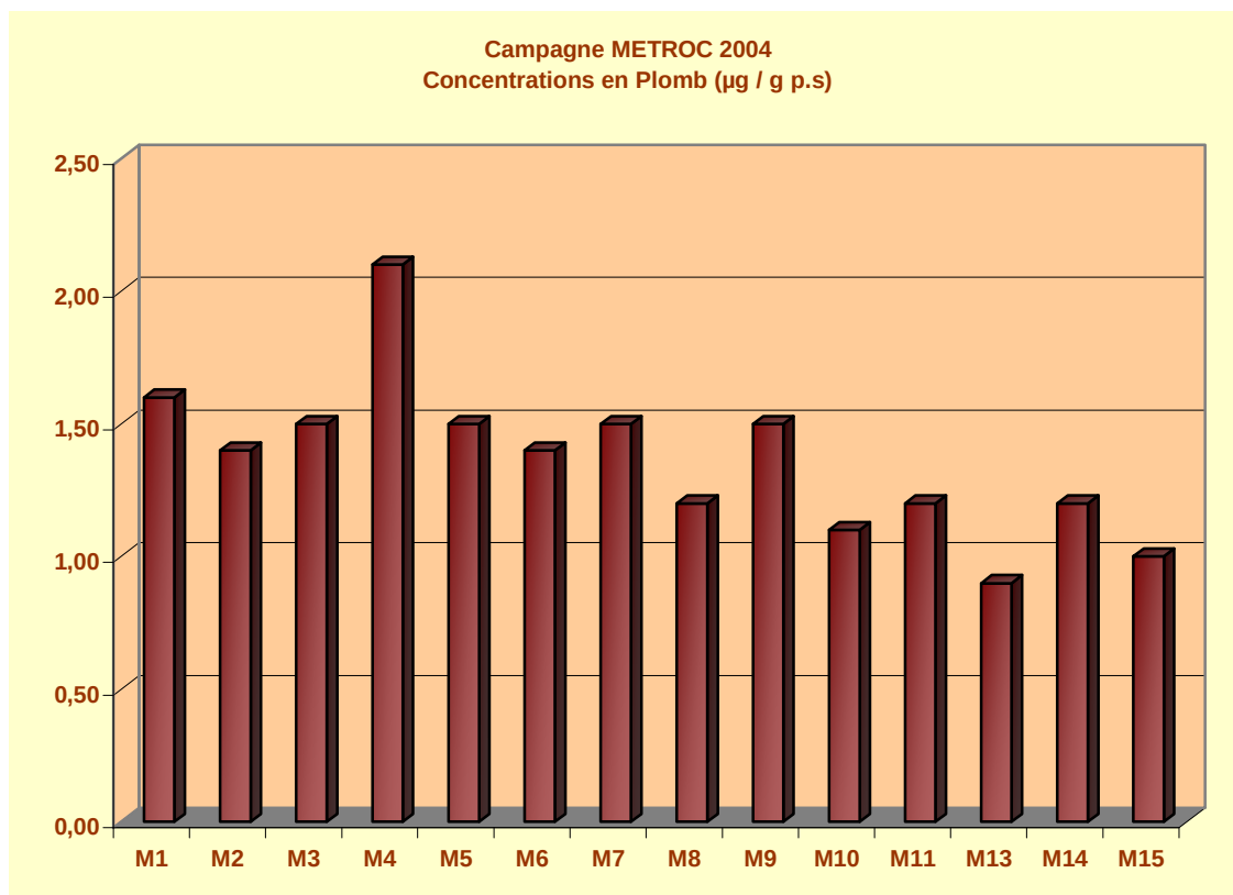
Figure 7 : Profils des concentrations en plomb mesurées dans le sédiment
