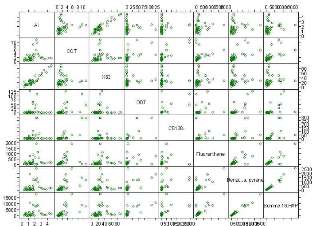
Figure 4 : Corrélations entre résultats de la campagne sédiment METROC 2004, les abscisses correspondent aux colonnes, les ordonnées aux lignes du tableau de graphes
